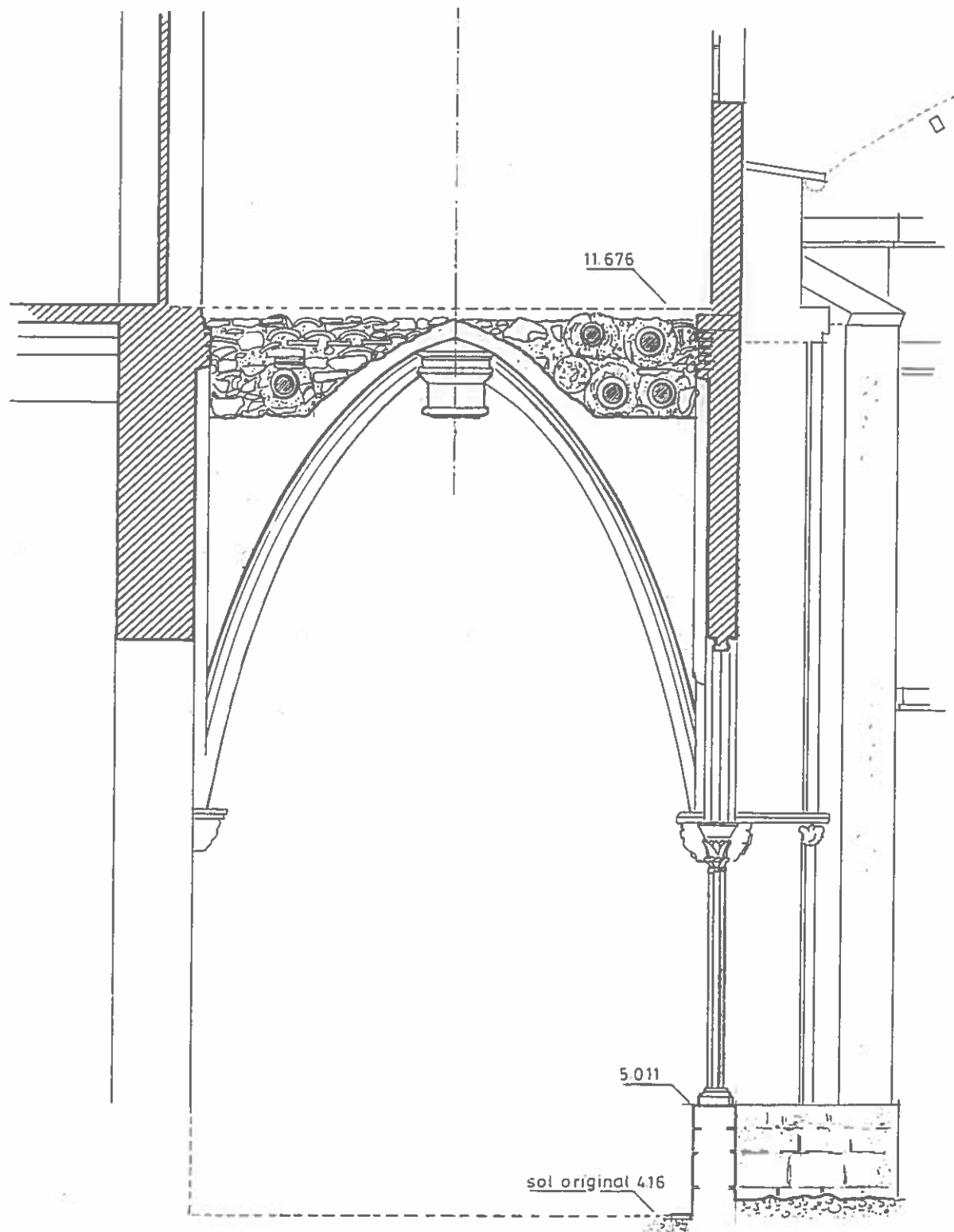
Secció transversal volta galeria.
